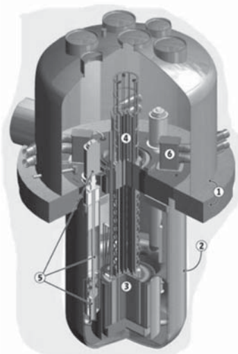
第8-17図 アモイ大学の進行波炉模型
