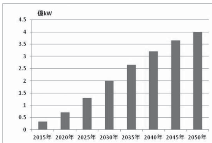
第8-3図 中国の原子力発電設備容量予測
