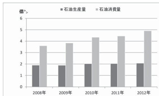
第5-21図 中国の石油消費量と生産量の推移
