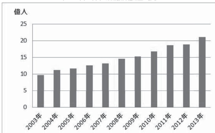
第7-10図 中国の鉄道旅客輸送量の推移
