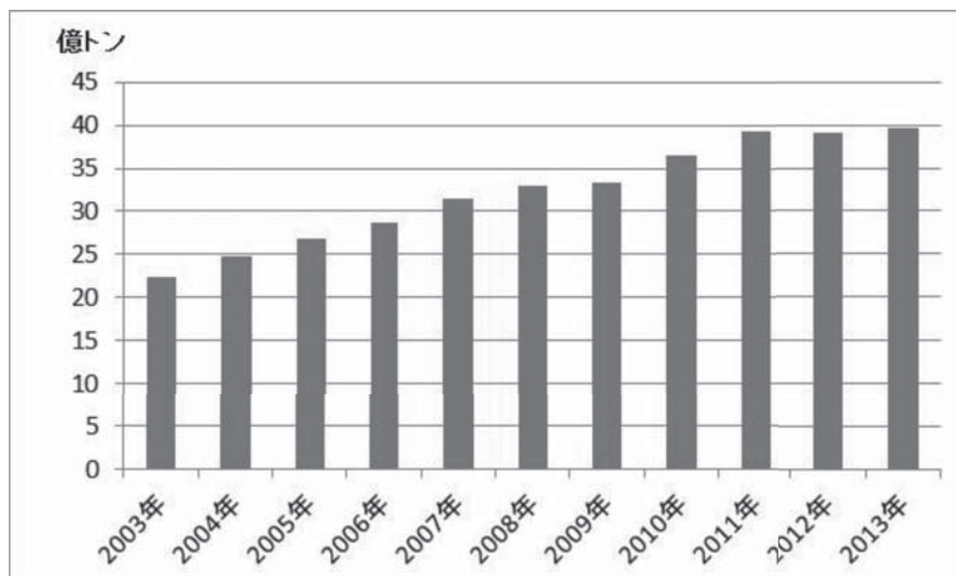
第7-11図 中国の鉄道貨物輸送量の推移
