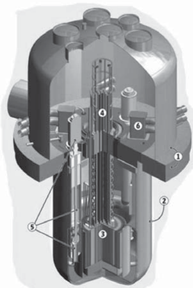
第8-17図 アモイ大学の進行波炉模型
